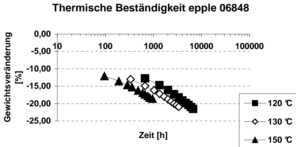
Abbildung 1: Gewichtsverlust (Prüfkörper 64 x 64 x 3 mm; Grenzwert 8 %)
