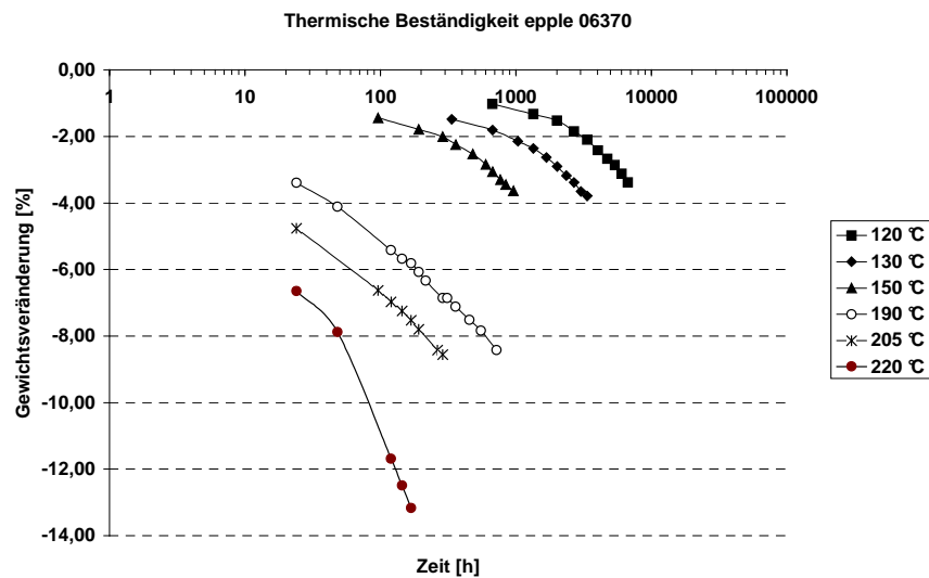
Abbildung 1: Gewichtsverlust (Prüfkörper 64 x 64 x 3 mm; Grenzwert 8 %)
